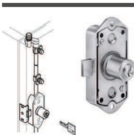
COD. GBW00003 SERRATURA CON ASTE ROTANTI con predisposizione chiave Passe-partout
